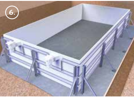
Liner en inbouwelementen installeren (skimmer, terugvoer)
