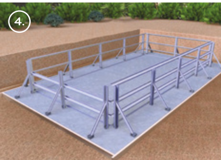
Plaatsing van de panelen (vastklikken + revetteren)
